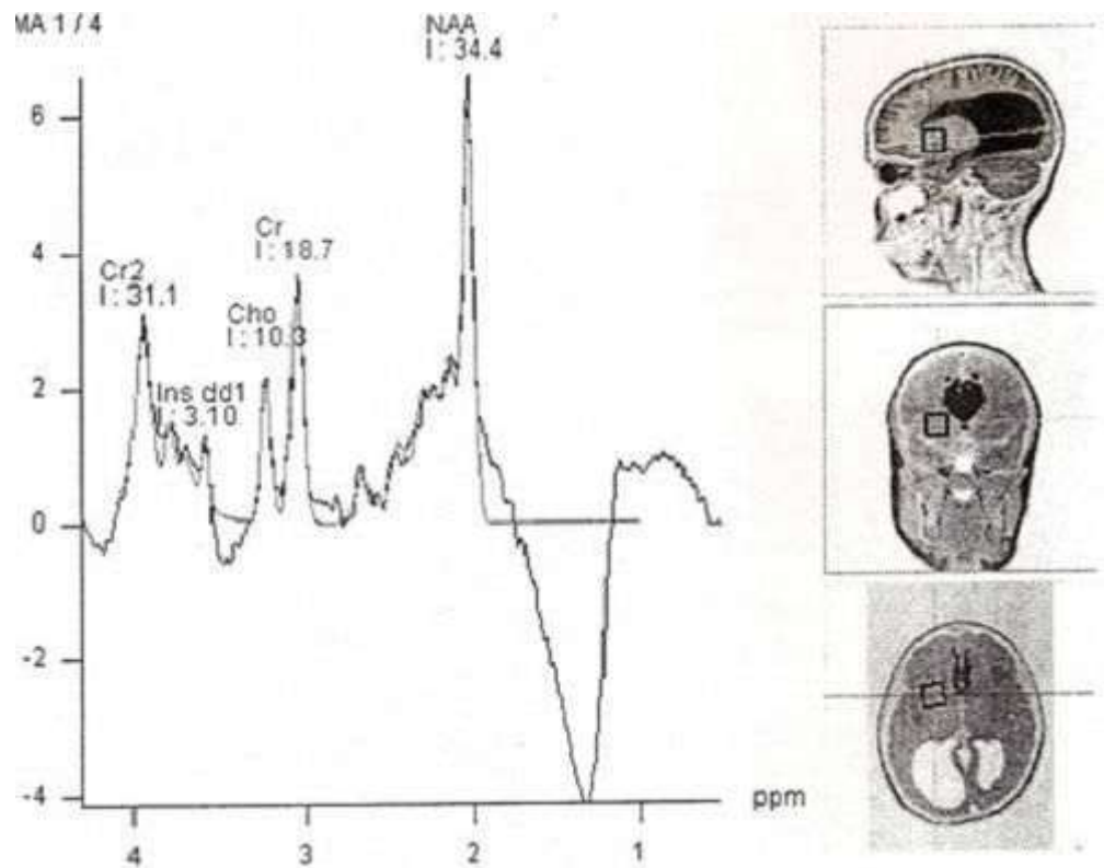
Fig. 6. Espectroscopia de H1 por Resonancia Magnética.
